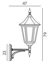
Art. 380 E27, 77W Halo. max. Black, 380B White, 380W EEI: A+..D
