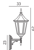
Art. 350 E27, 77W Halo. max. Black, 350B White, 350W EEI: A+..D
