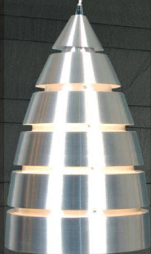
MDE135/1CLI Ø26,00 × 41,00 E27 1 × 60W
