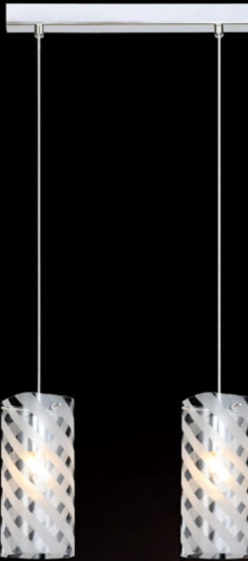
MDM2044-2 32,00 × 10,00 × 100,00 E27 2 × 60W
