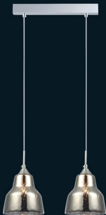
MDM2387/2 SG 38,00 × 16,00 × 100,00 ⦿ E14 2 × 40W
