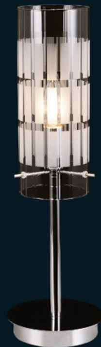
MTM1957-1 Ø14,00 × 46,00 E27 1 × 60W
