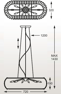
ANTARCTICA Pendant P0174-10A 10*G9 42W MAX K9 clear crystal / metal chrome
