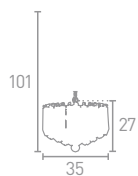
F 6715CC Chrome/Acrylic 4x60w E14
