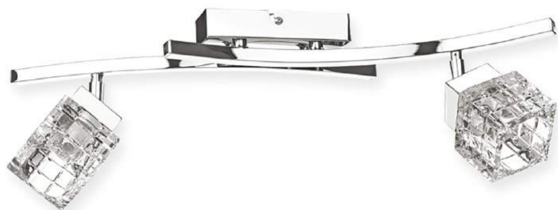
O1982 P2 CH → 56 x 13 cm ↓ 13-20 cm 2 x E14 max 60W
