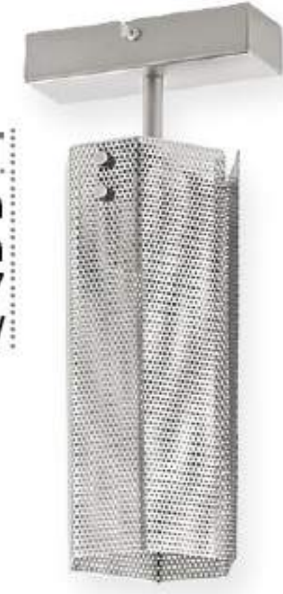
O1787 SAT ↔ 15 x 10 cm ↓ 33 cm 1 x E27 max 60W
